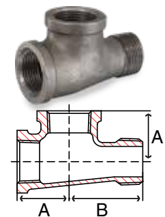
Fig. 33ST1 & 34ST1 – Service Tee
